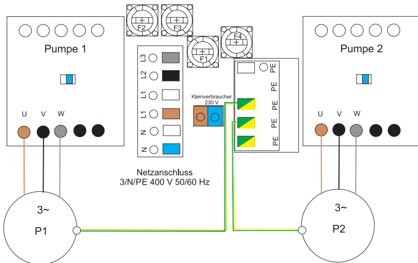
Anschluss 3-Phasen Motor
