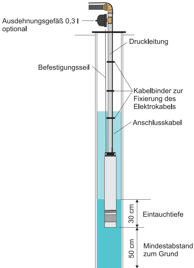
Montageskizze für die AQUASTREAM 50 im Brunnen
