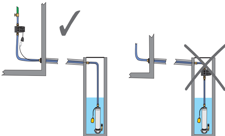
Anwendungsbeispiel mit Tauchpumpe
